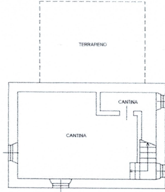
PIANO SOTTOSTRADA 1 (SEMINTERRATO) H. 2.40
