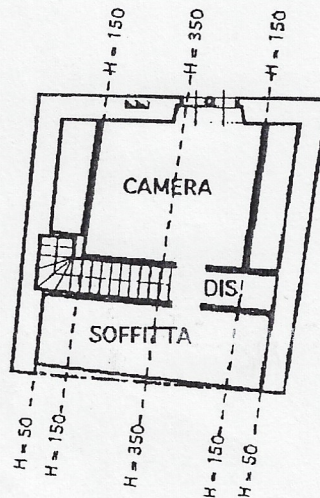
PIANO SECONDO (SOTTOTETTO)
